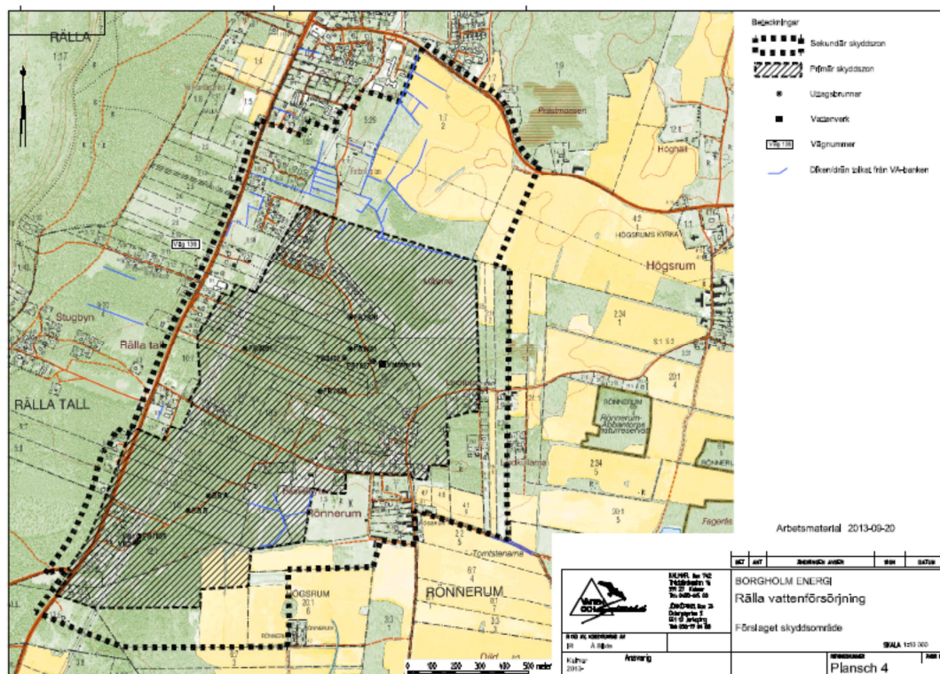
Fig 1. Förslag på nytt vattenskyddsområde för Rälla vattentäkt (Vatten och Samhällsteknik, 2013)
