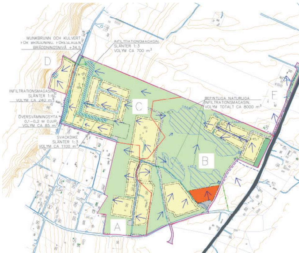
Bild 5. Dagvattenhanteringsplan för Stora Rör 2:1 m.fl. Naturliga infiltrationsytor illustreras i öst och anlagda ytor i väst. Planförslaget har justerats efter att utredningen togs fram men principen för dagvattenhantering är densamma även efter justering.
