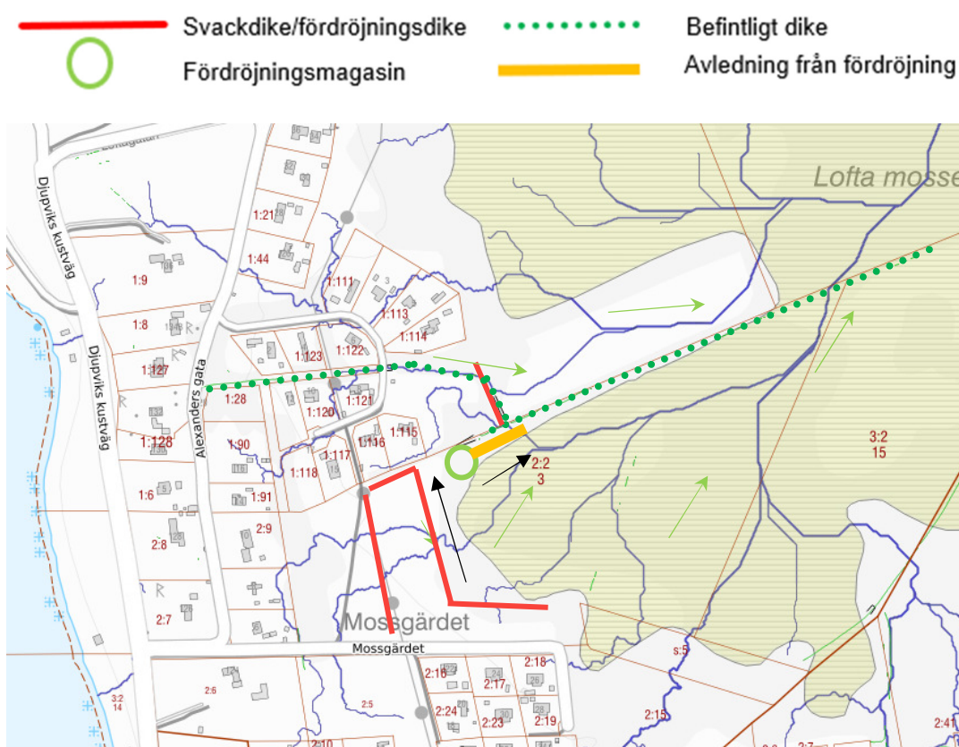
Figur 15: Ytliga flödesvägar samt planerad dagvattenhantering.
