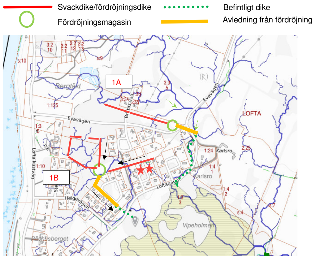
Figur 9: Ytliga flödesvägar samt planerad dagvattenhantering. Översvämningsdrabbade fastigheter markerade med röd stjärna.
