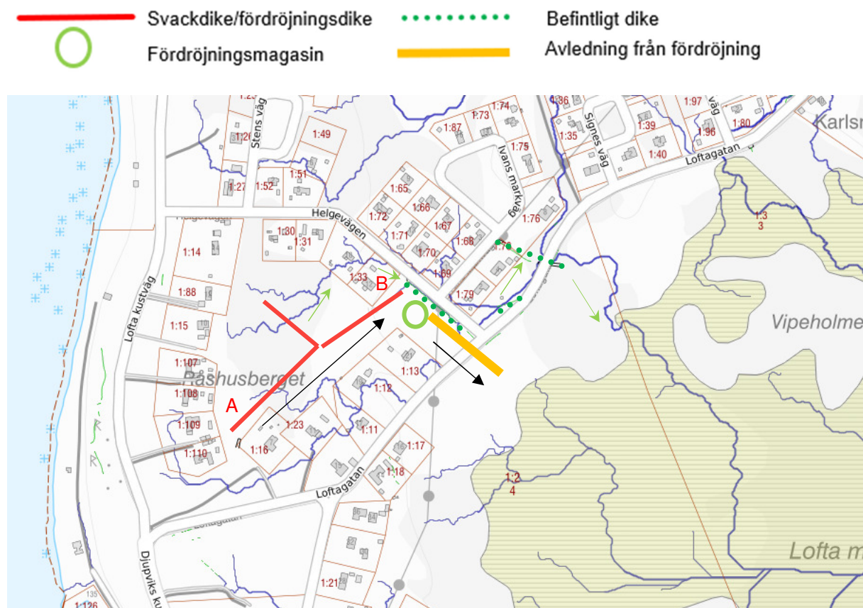
Figur 12: Ytliga flödesvägar samt planerad dagvattenhantering.
